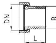
Фитинги резьбовые
