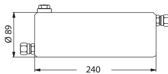
Охладитель импульса давления V1
