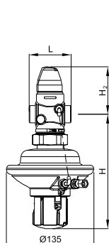
AVPQ DN = 15–50 мм, \Delta P_{рез} = 0,2–1,0 бар
