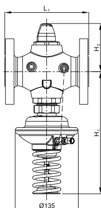
AVPQ DN = 32–50 мм, \Delta P_{рез} = 0,3–2,0 бар
