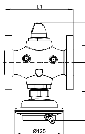
AVPB-F DN = 32–50 мм
